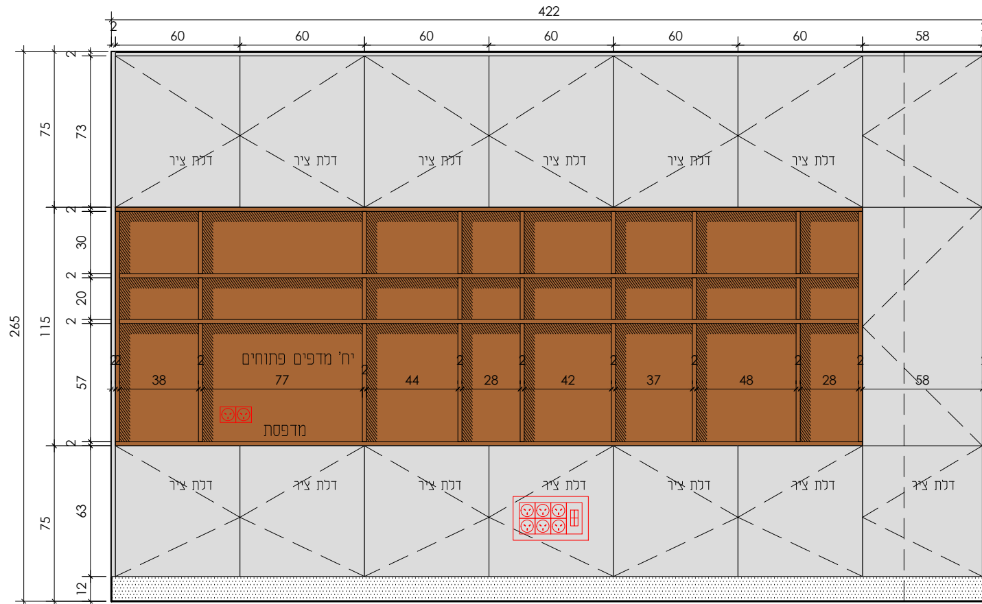
חזית קנ"מ-1:20
